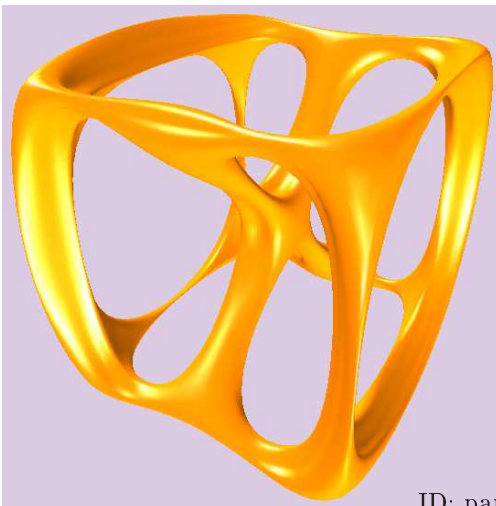
(d) Interpolating Surface
